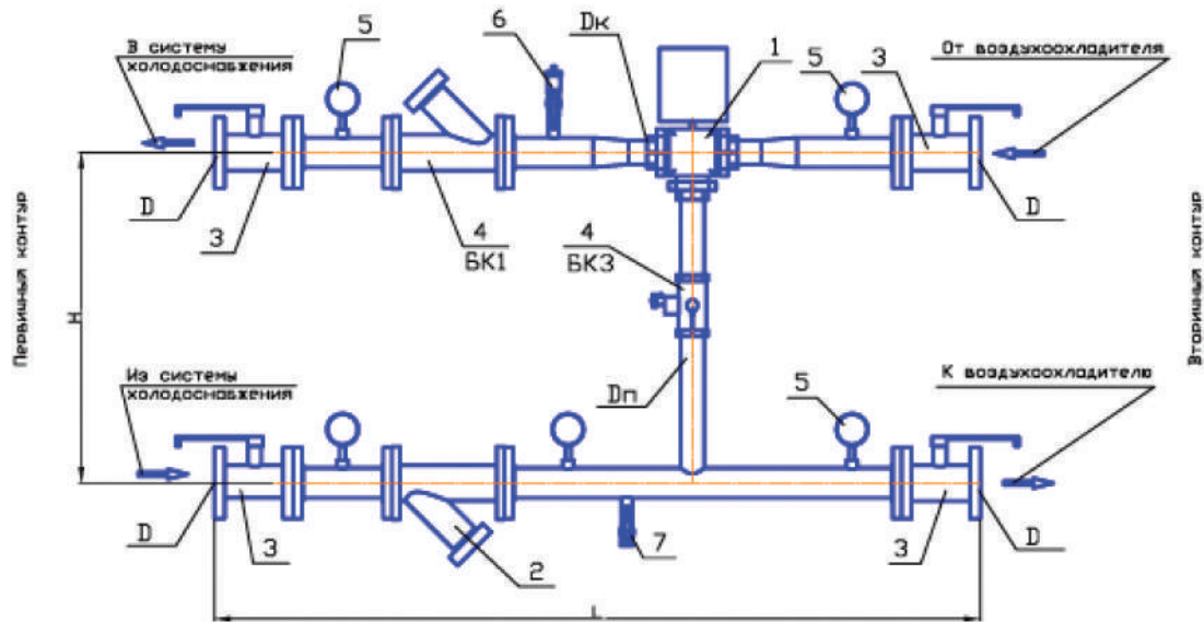
Узел регулирования УР2
