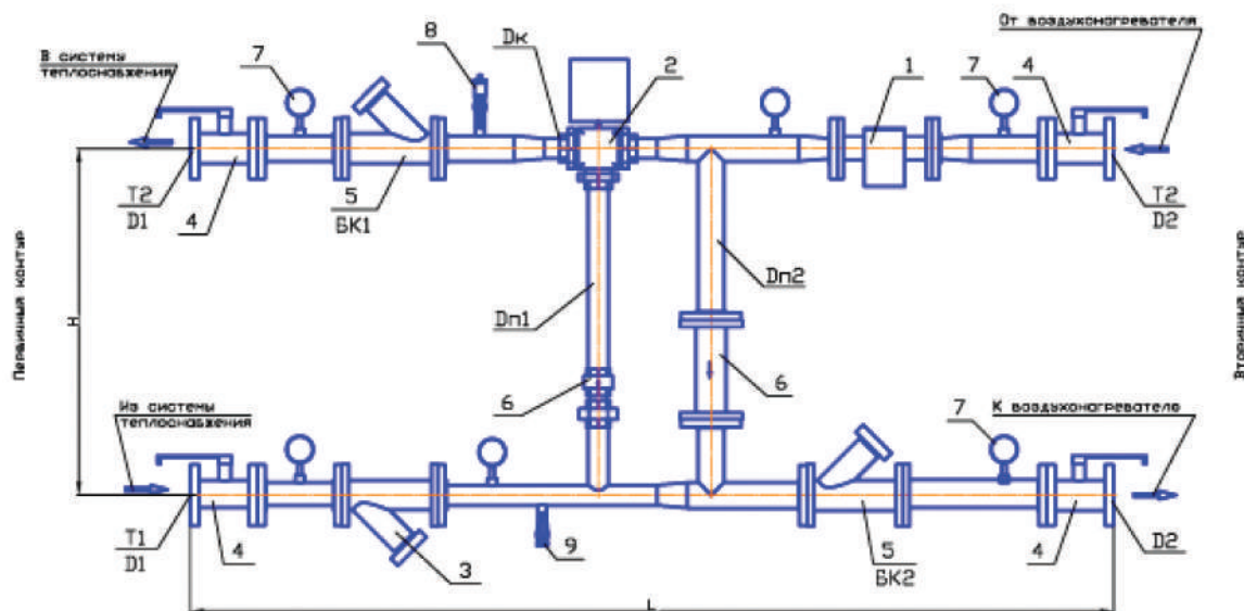
Узел регулирования УР1.2
